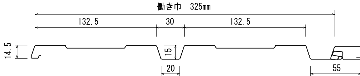
リブタイプ
