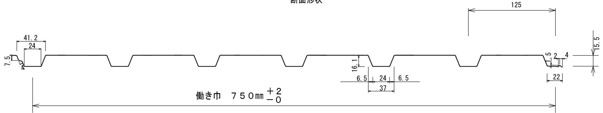
断面形状
