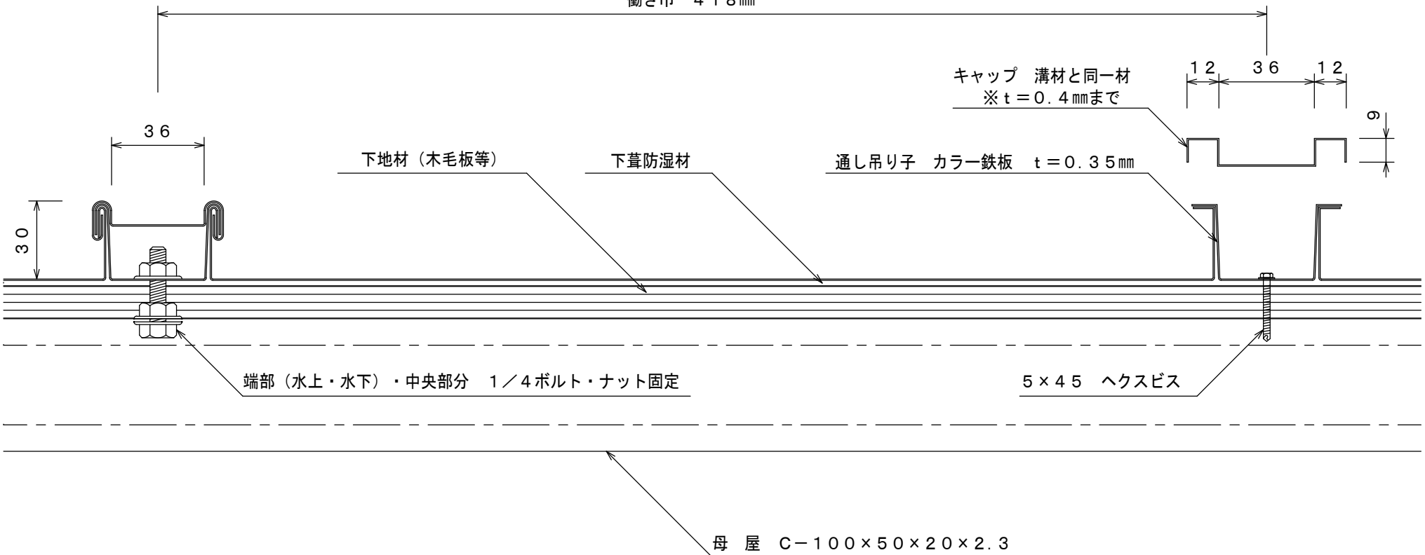
溝板寸法
