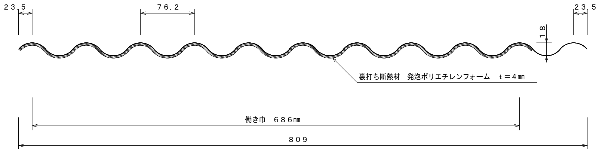
断面形状
