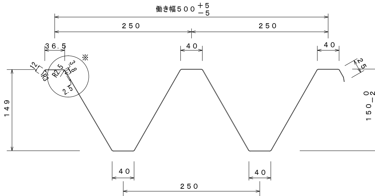
断面形状
