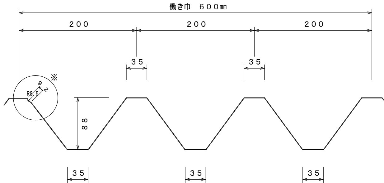
断面形状
