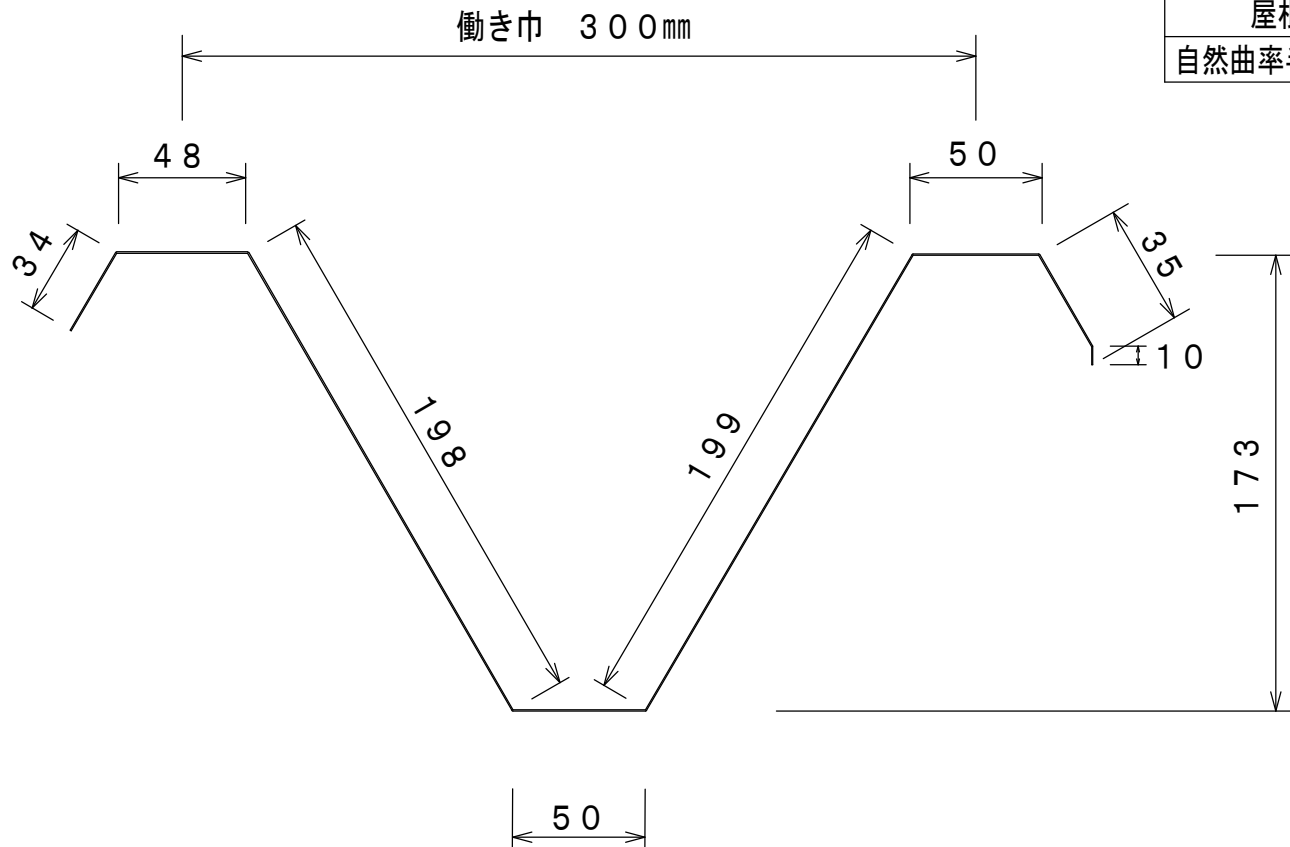
断面形状
