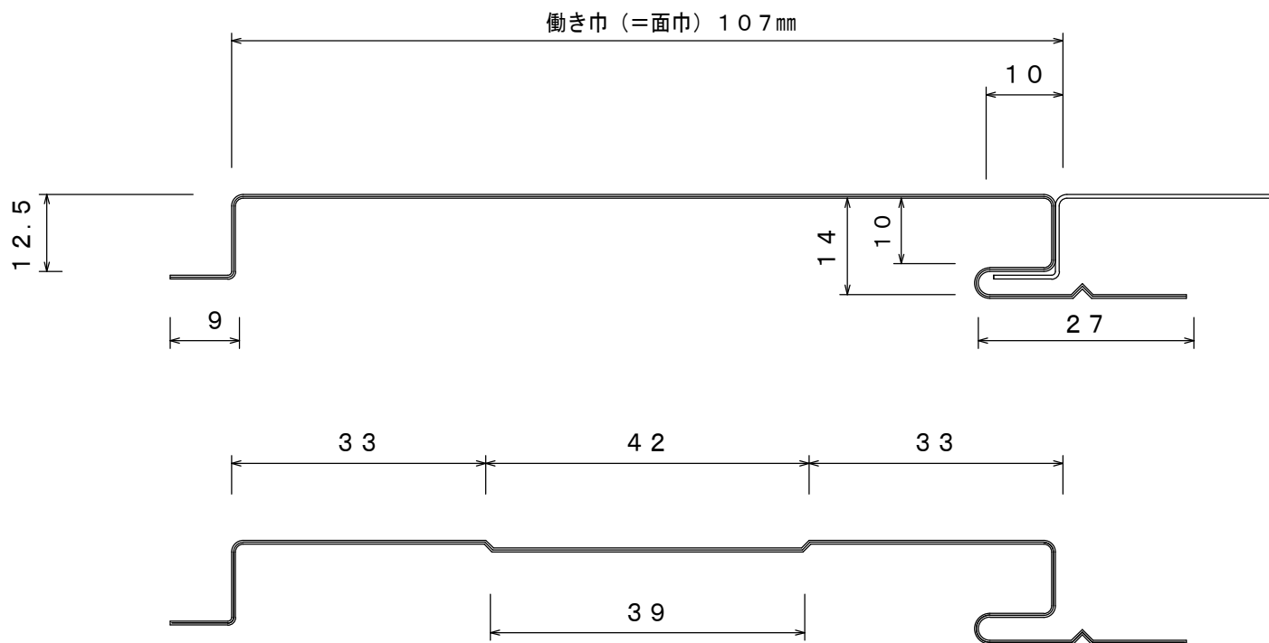
断面形状
