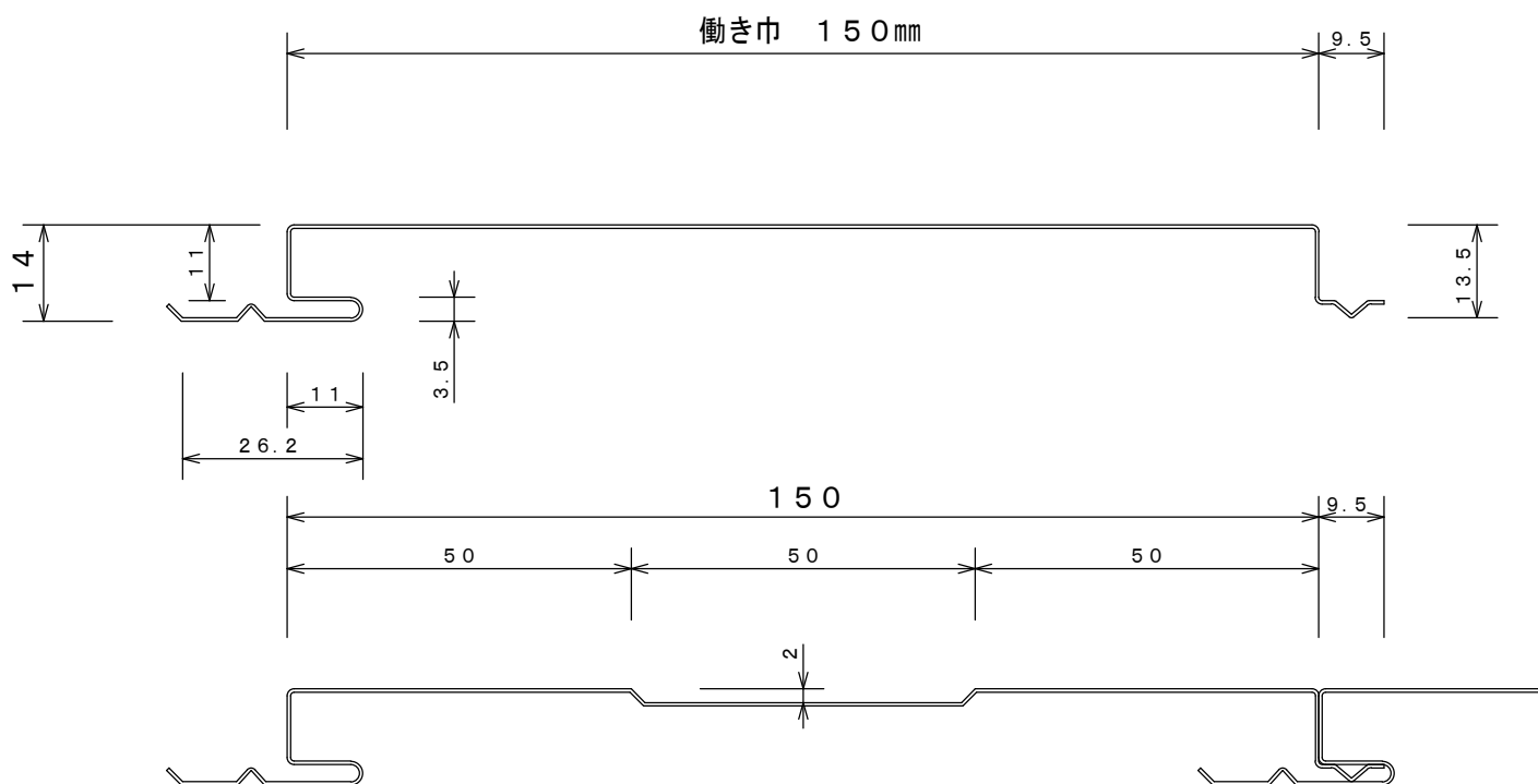
断面形状
